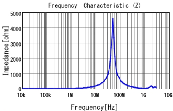
■ 1217AS-H-3R3N |Z|
