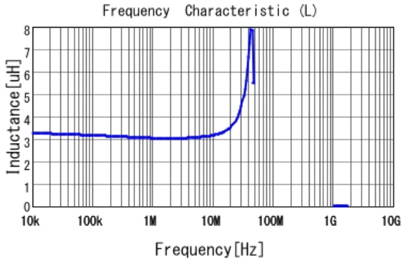
■ 1217AS-H-3R3N L
