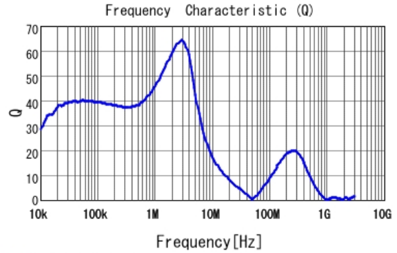
■ 1217AS-H-3R3N Q
